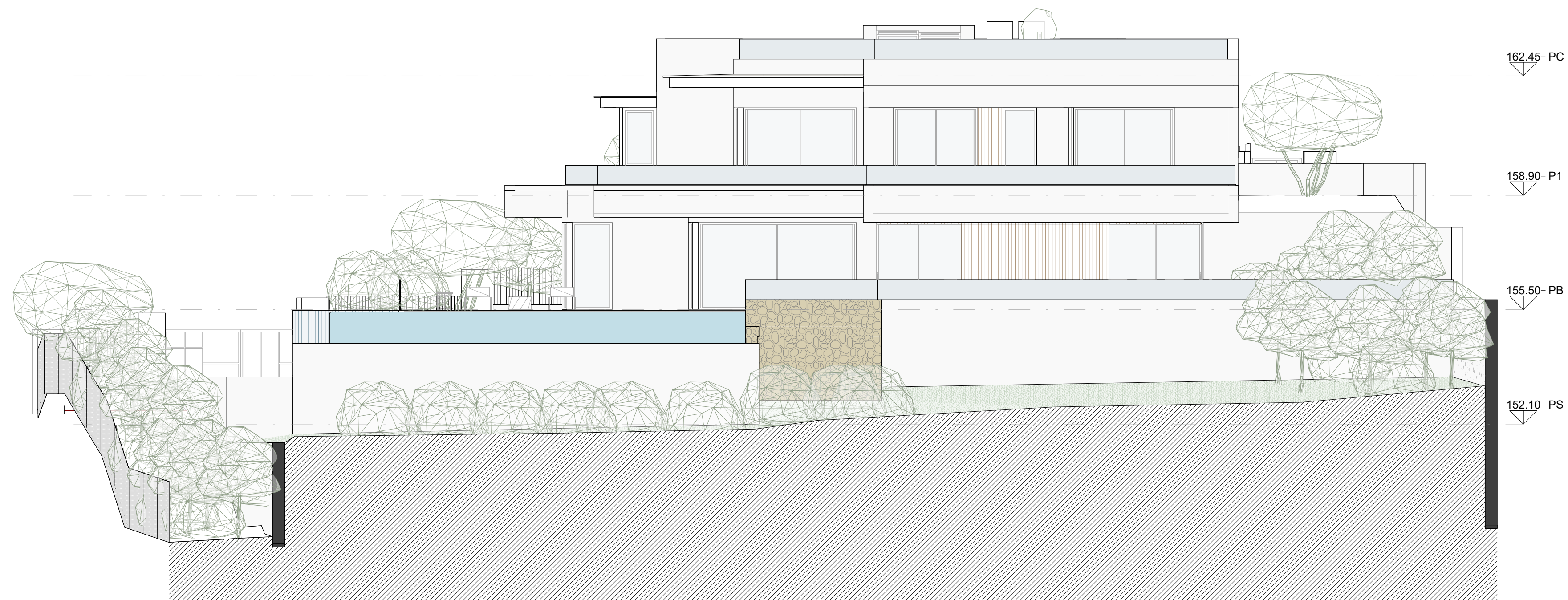
Elevation
